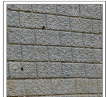
E-127 布紋砌 單元尺寸 91.5 x 45.7 x 4.5 cm
